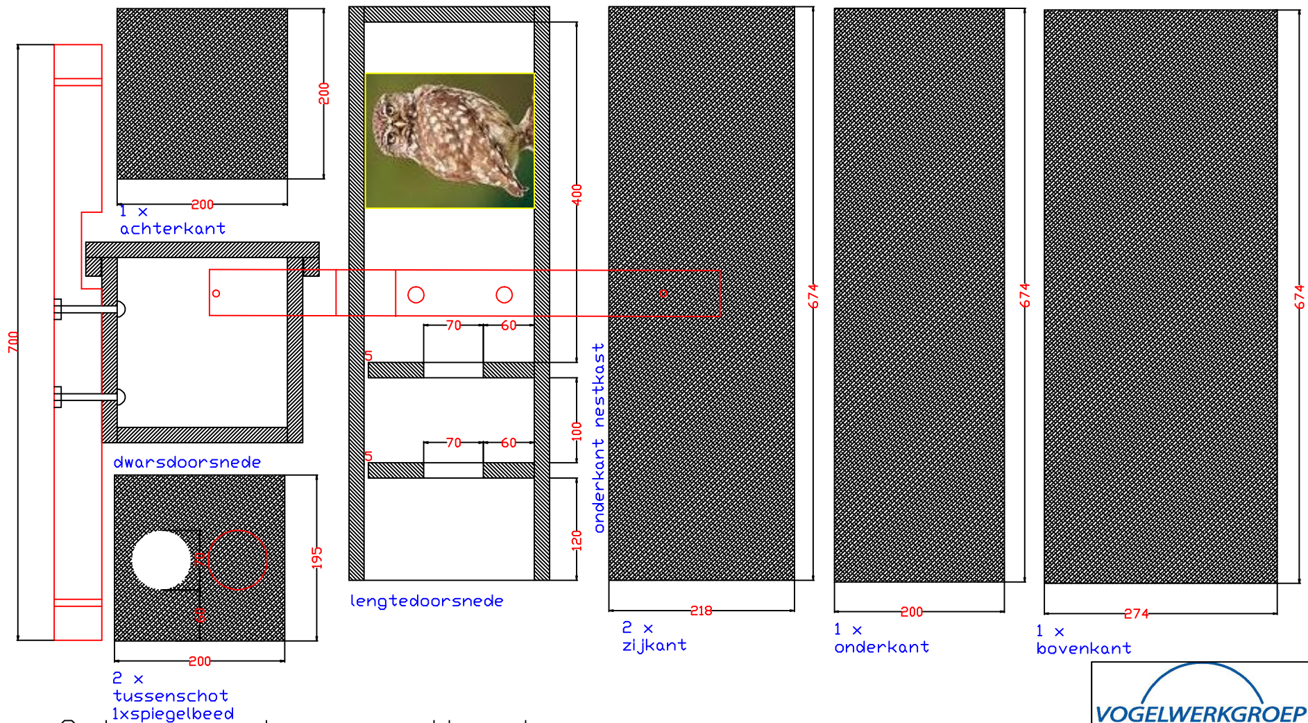
Schema opbouwnestkast steenuil met maatvoering
